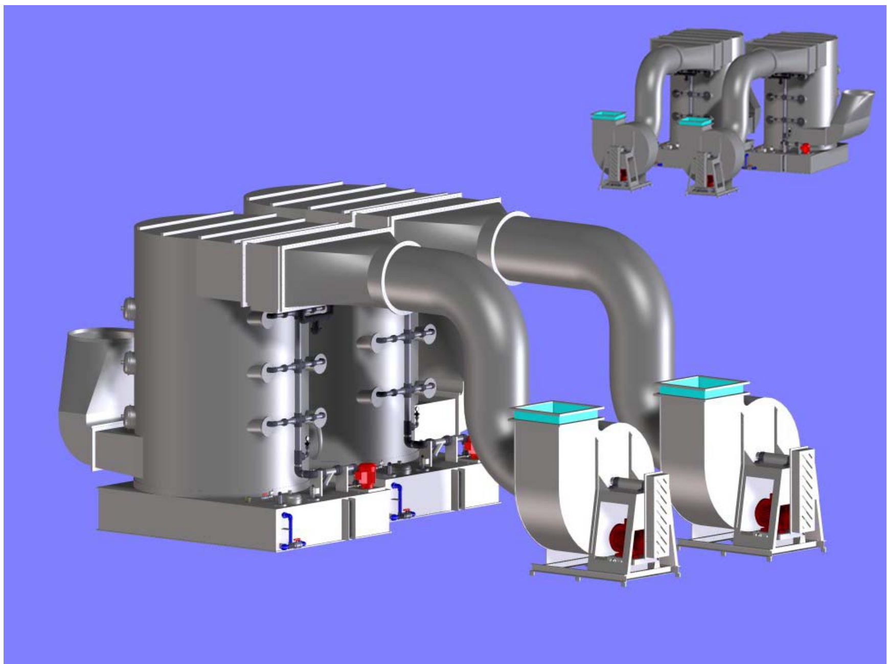
Kraftwerksausrüstung. Abluftreinigungsanlage für 40.000 m 3 /h Abluft mit angeschlossenen Ventilatoren VR 900-56 RMU
